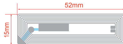
天线图 (Antenna)
